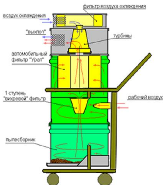
Рис. 2. Структурная схема работы пылесоса
