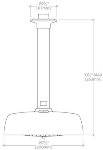
SIDE VIEW SCALE: 3"=1'-0"
