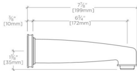
SIDE VIEW SCALE: 3"=1'-0"
