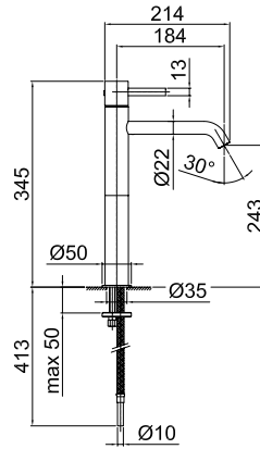
ART. A706WF Gruppo lavabo / Washbasin / Lavabo 1 trous / Waschtischarmatur / Lavabo
