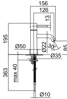
ART. A704WF Gruppo lavabo / Washbasin / Lavabo 1 trous / Waschtischarmatur / Lavabo
