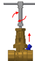
3. Introducir la llave especial hasta enganchar el tornillo y girar en sentido horario hasta que el accionamiento salga del tope del cuerpo hacia arriba. / Insert the special key to engage the screw and rotate clockwise until the handle go out the body's stop upward.
