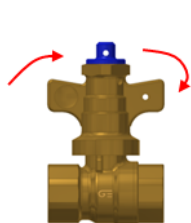
1. Interrumpir el flujo del agua girando el accionamiento en sentido horario. / Stop the water flow rotating the handle in clockwise.
