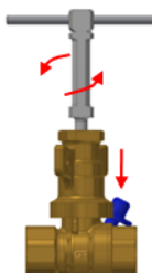
5. Introducir de nuevo la llave especial hasta enganchar el tornillo y girar en sentido anti-horario. El accionamiento quedará bloqueado y no se podrá girar. / Fit the special key again, engage the screw and rotate counter-clockwise. The handle will remain locked and you can not rotate it.
