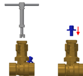
6. Extraer la llave e introducir el tapón de protección. La válvula permanecerá bloqueada (en 10% apertura). / Remove the key and insert the plastic protection cap. The valve will remain locked (at 10% opening).
