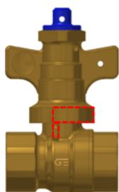
A) Función normal Abrir / Cerrar manualmente A) Normal function Open / Close manually
