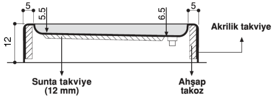
Kesit A-A
