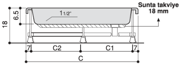
Kesit A-A
