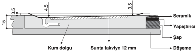
Kesit A-A
