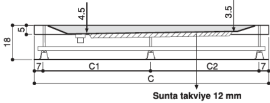
Kesit A-A
