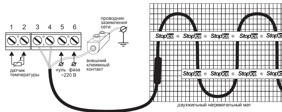
Рис. 2. Схема подключения нагревательного мата МНТ2 к терморегулятору TP 140
