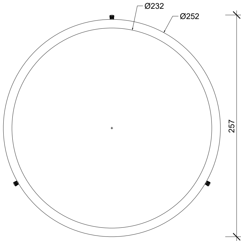
Untersicht bottom view
