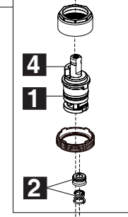
RP74418 Stem Unit Assembly, Seat & Spring, Bonnet Nut & Washer Ensamble de la Unidad del Vástago, Asiento y Resorte, Bonete y Arandela Obturbador, siège et ressort, écrou à chapeau et rondelle
