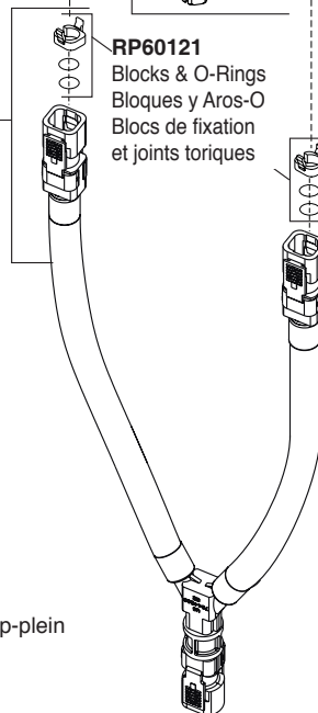
RP100526 Hose Assembly, Blocks & O-Rings Ensamble de la manguera, Bloques y Aros-O Tuyau souple, blocs de fixation et joints toriques
