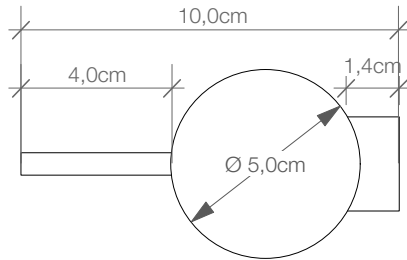
Draufsicht Top view
