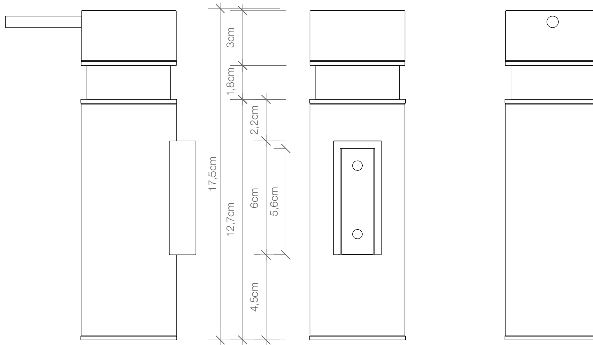
Seitenansicht Side view
