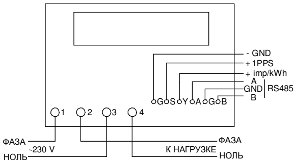
Схема подключения счётчиков НЕВА МТ 11Х
