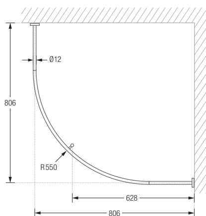
Produktbeispiel DSB550-800K45 Draufsicht:
