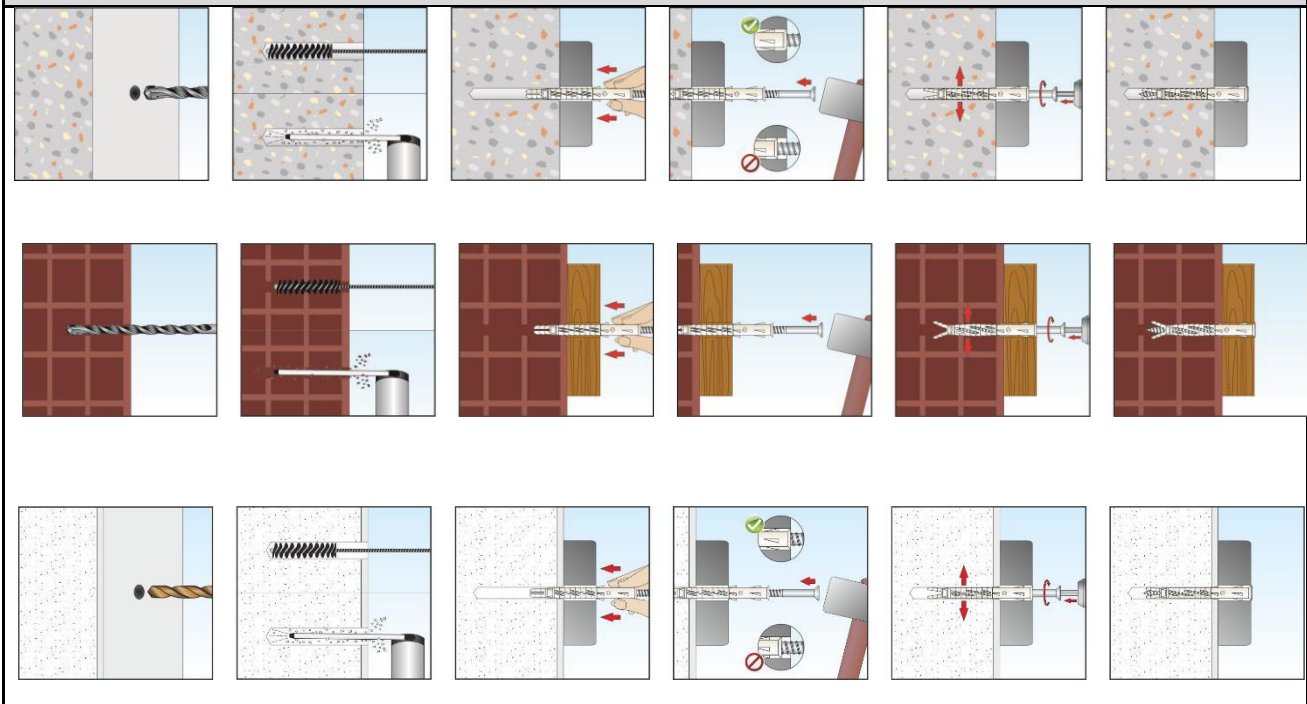
Figura 2 - Sequenza d'installazione
