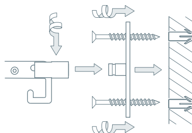
Montage mit ovaler Rosette:
