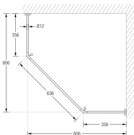
Produktbeispiel DSFE800K45 Draufsicht:
