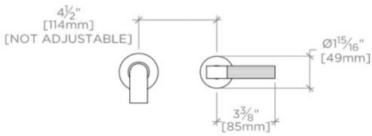
TOP VIEW SCALE: 1/2"=1'-0"
