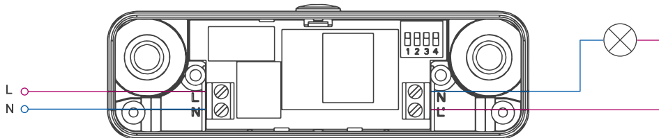
Рисунок 3. Схема подключения датчика движения.
