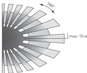
Рисунок 2. Схема зоны обнаружения.
