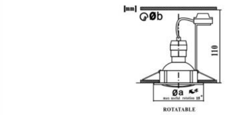
ROTATABLE
