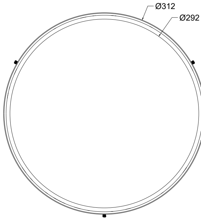
Untersicht bottom view
