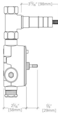
SIDE VIEW SCALE: 3"=1'-0"
