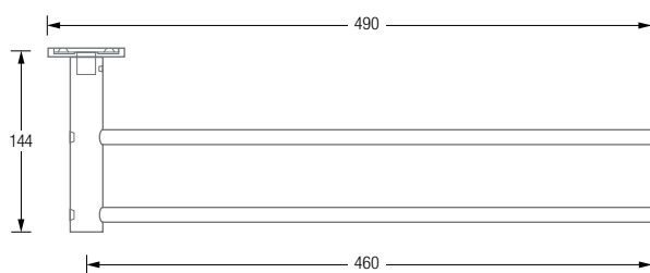
HS26-140EDS460 Draufsicht:
