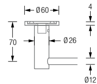
HS26-140EDS460 Detailansicht:
