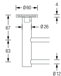
HS26-140EDS460 Detailansicht:
