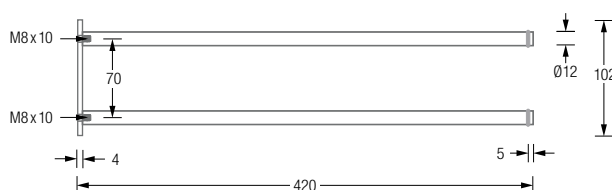
Produktbeispiel HS12-420D-0 Draufsicht:
