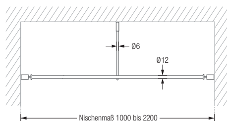
Produktbeispiel DSGN12-2 Frontansicht:
