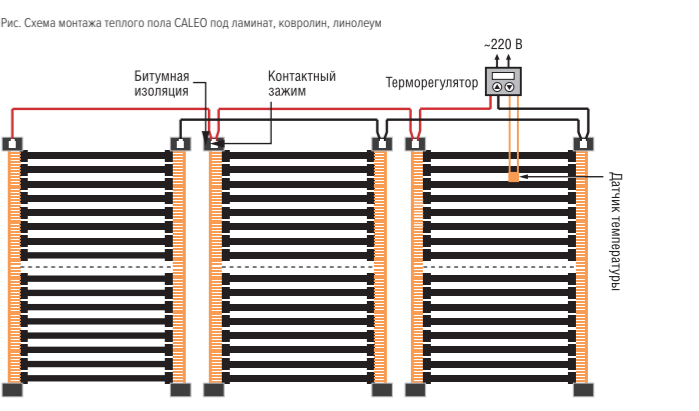
Рис. Общая схема подключения термопленки CALEO
