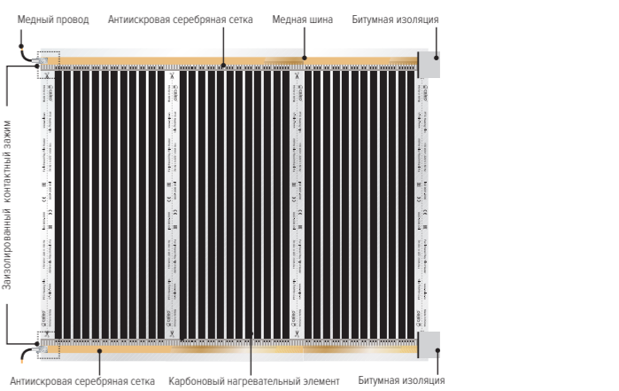
Рис. Общий вид термопленки CALEO, расположение основных ее элементов, контактных зажимов и мест подключения и изоляции
