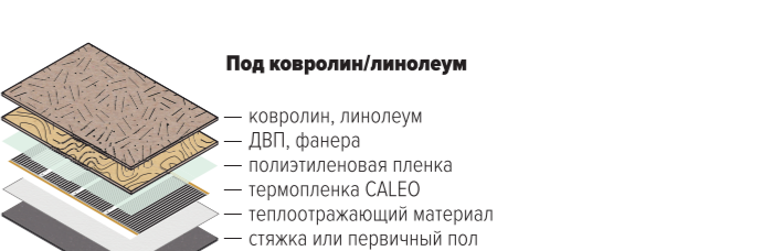
Рис. Схема монтажа теплого пола CALEO под ламинат, ковролин, линолеум
