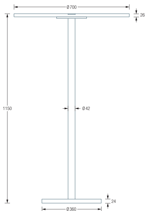
T1150-Eiche Seitenansicht:
