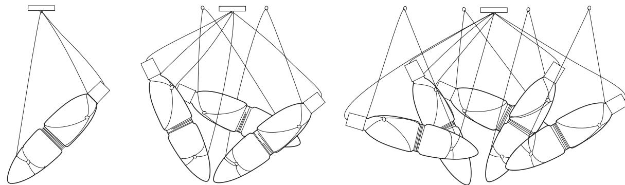
pendant 1 position →← 450 ↑↓ 600 pendant 3 position →← 550 ↑↓ 750 pendant 5 position →← 900 ↑↓ 950
