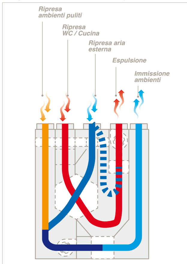
Funzionamento in deumidificazione e integrazione con rinnovo aria e parziale ricircolo
