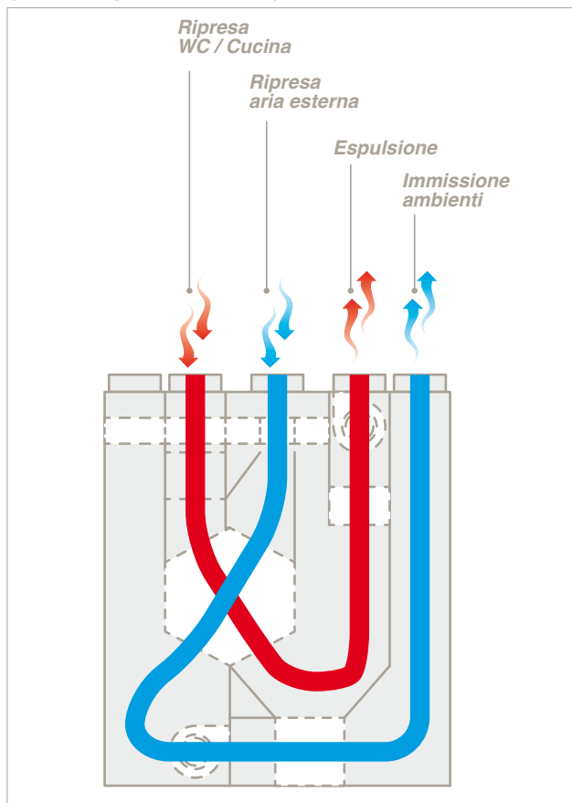
Funzionamento in solo rinnovo aria ambiente (ad esempio in inverno)
