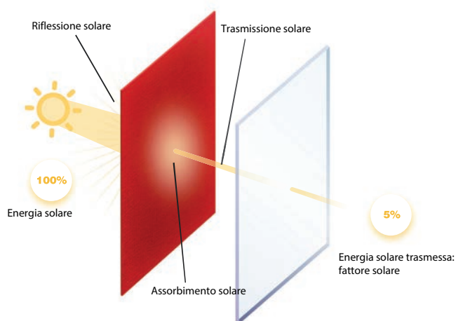
Protezione esterna con Soltis Perform 92-2045 (cfr. Guida Design)
