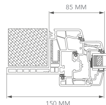
NODO LATERALE Side mullion / Meneau latéral
