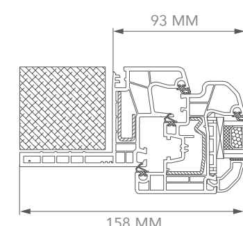
NODO LATERALE Side mullion / Meneau latéral
