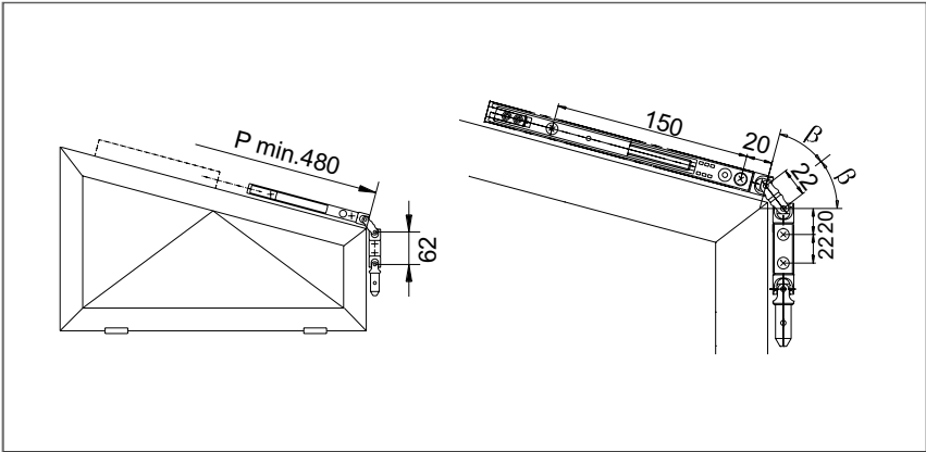
Finestre inclinate con Fz 92
