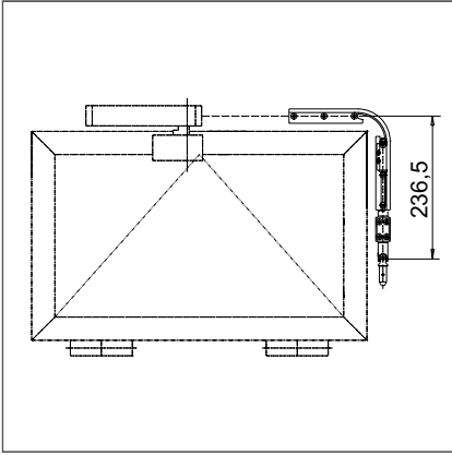
Finestre rettangolari con GEZE Fz 100
