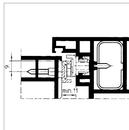
FPS su finestre in materiale sintetico
