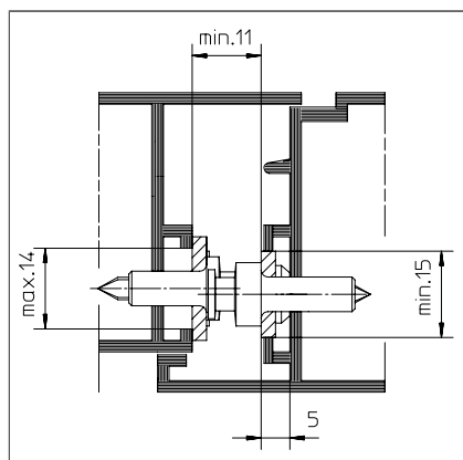
FPS su finestre in lega leggera (montaggio senza spessori)
