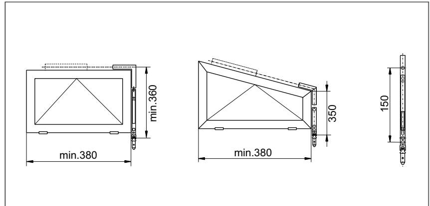
Finestre rettangolari e inclinate con GEZE Fz 91
