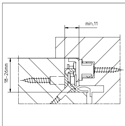
FPS su finestre in legno
