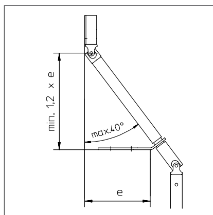
Disegno di installazione pendolo Biella fissa e = profondità telaio
