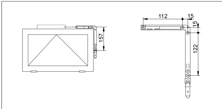
Finestre rettangolari con GEZE Fz 90
