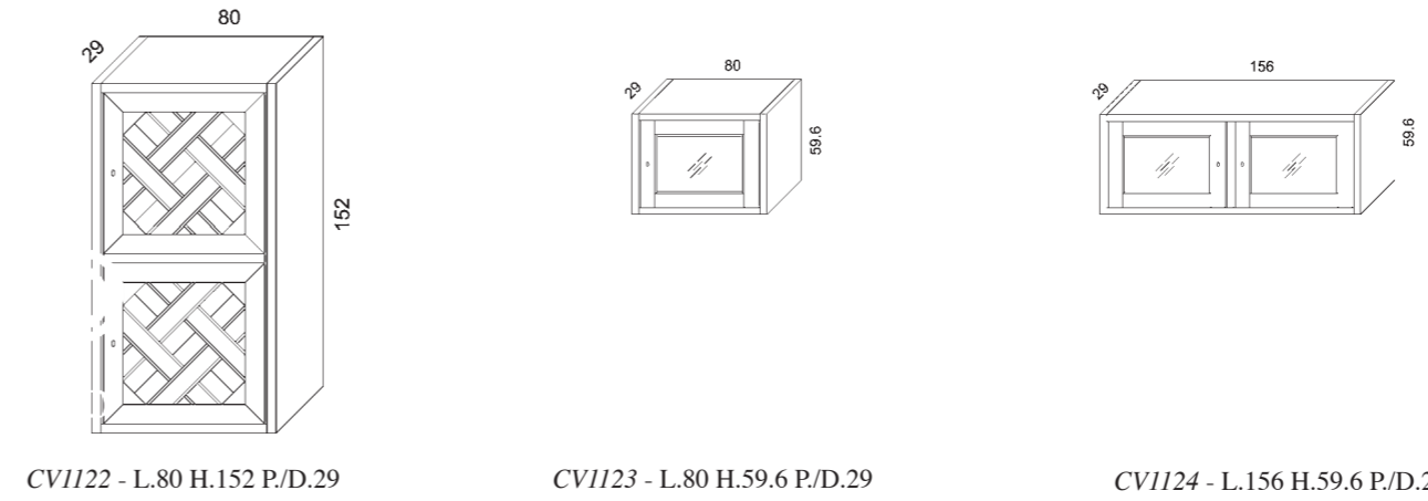
CV1122 - L.80 H.152 P/D.29 CV1123 - L.80 H.59.6 P/D.29 CV1124 - L.156 H.59.6 P/D.29
