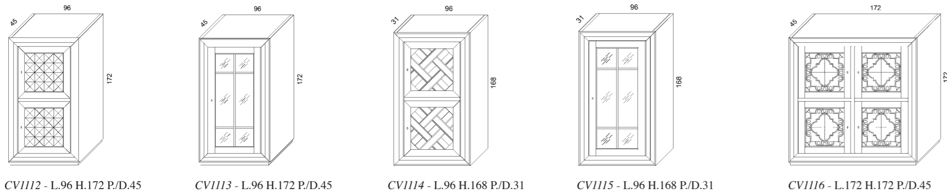
CV1112 - L.96 H.172 P/D.45 CV1113 - L.96 H.172 P/D.45 CV1114 - L.96 H.168 P/D.31 CV1115 - L.96 H.168 P/D.31 CV1116 - L.172 H.172 P/D.45
