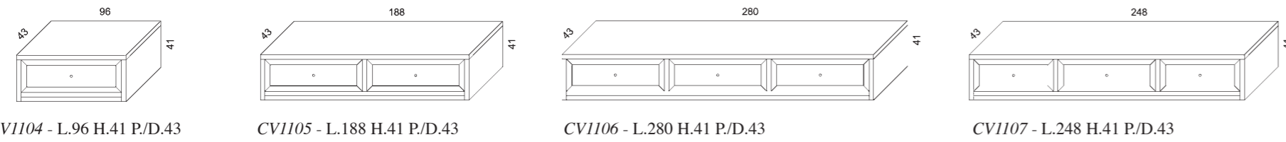
CV1104 - L.96 H.41 P/D.43 CV1105 - L.188 H.41 P/D.43 CV1106 - L.280 H.41 P/D.43 CV1107 - L.248 H.41 P/D.43
