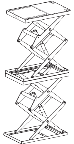
quadruplo pantografo
